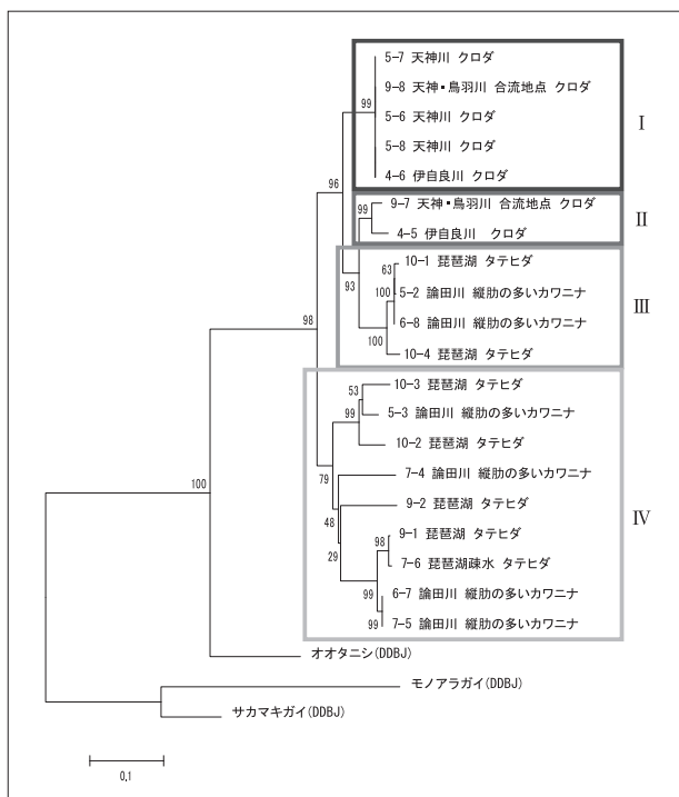
図16 分子系統樹
