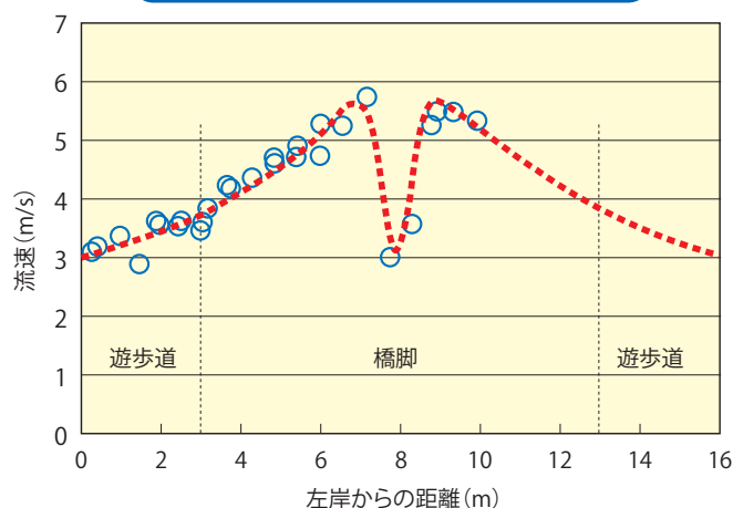
橋脚下流の横断表面流速分布
