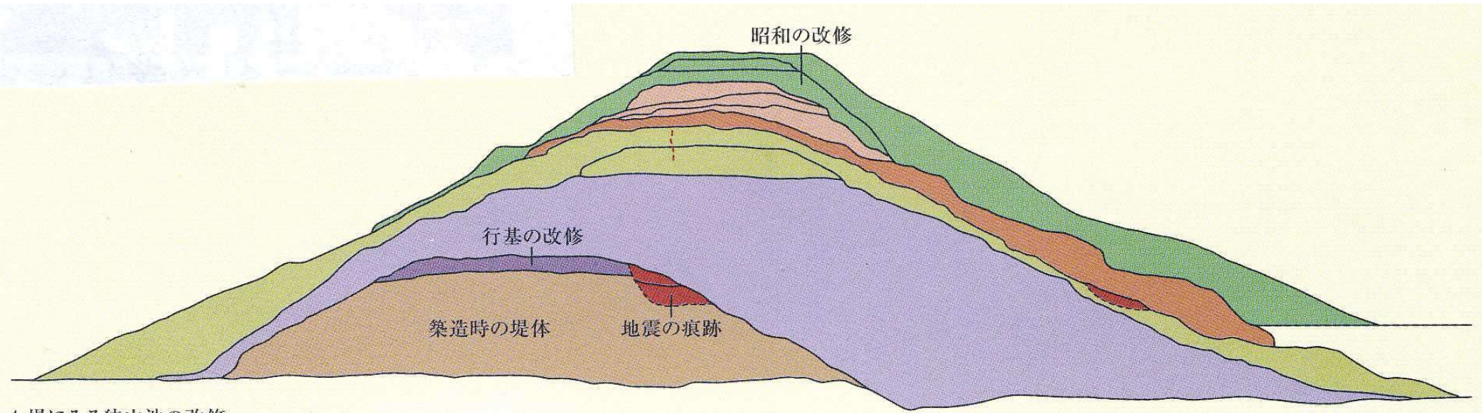
4 堤にみる狭山池の改修
